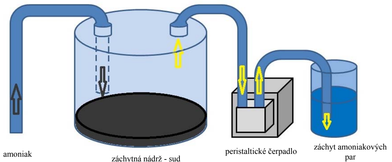
Nákres zapojení podtlakového sběrače
